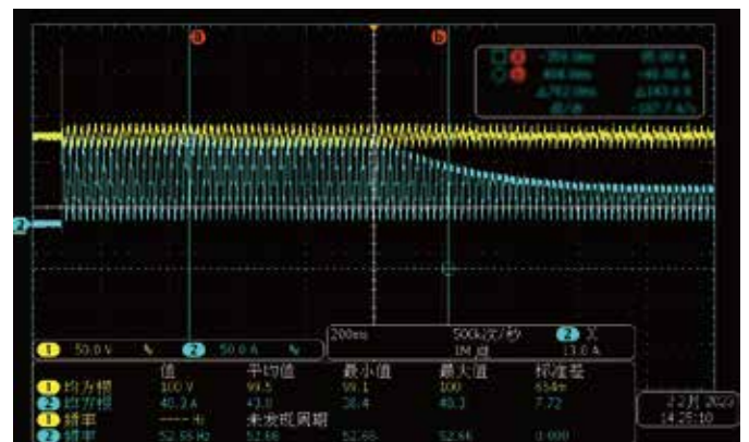
AC+DC模式, AC20A+ DC30A, 50Hz; 限电流10A, 进入电流环
