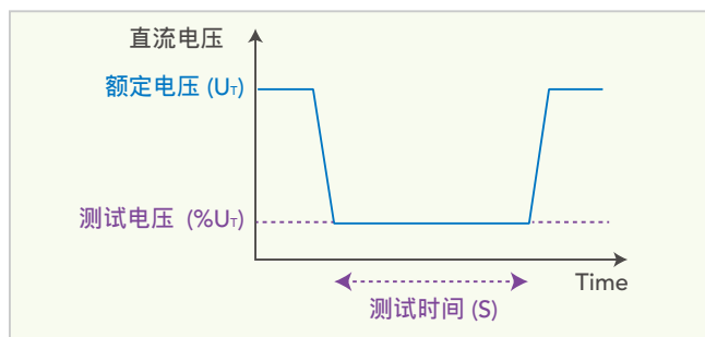
直流输入电压抗扰度测试
