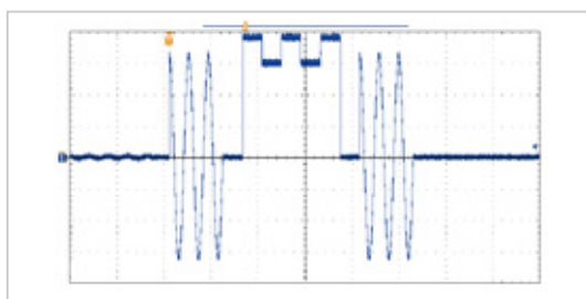
61509实际输出电压波形
